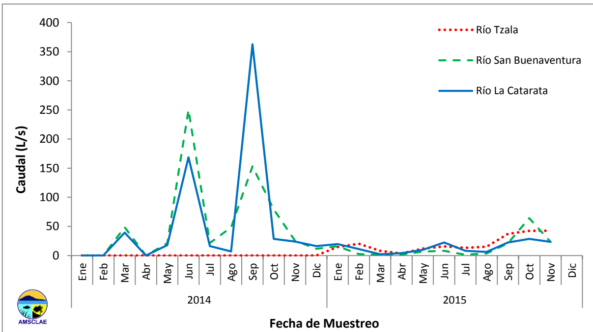
Figura 2. Variación temporal general de caudales (L/s) de los principales ríos tributarios de la Cuenca del Lago de Atitlán, durante el 2014 y 2015 (AMSCLAE/DICA, 2015)
